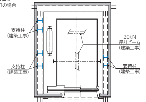
支持柱設置の場合
