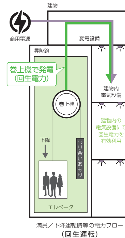
満員/上昇運転時等の電力フロー (力行運転)
