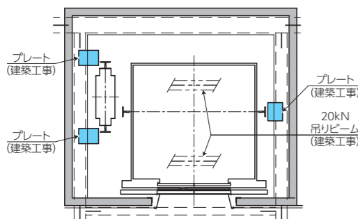
P 乗用据付図④
