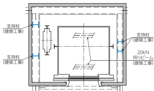
P 乗用据付図④
