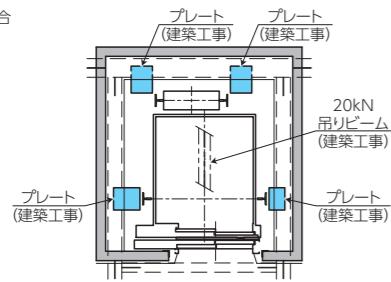
プレート設置の場合
