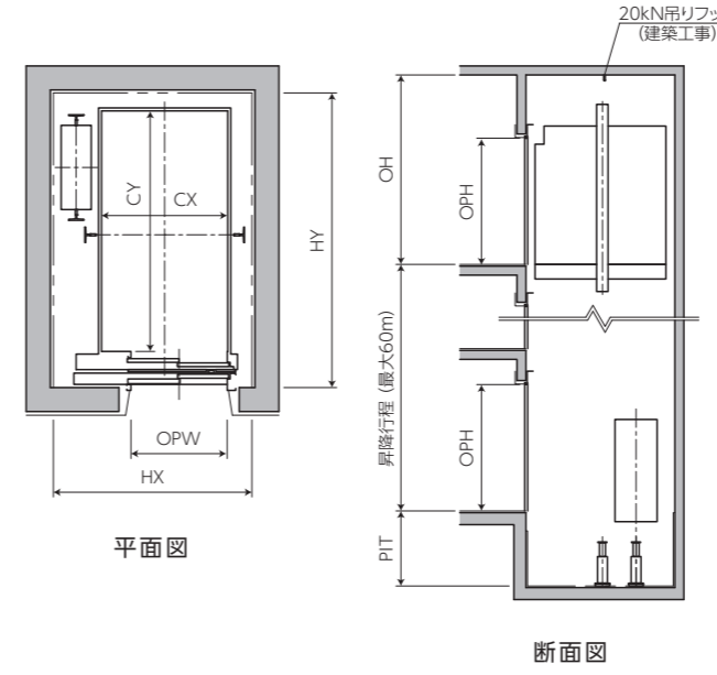
一方向出入口据付図
