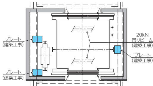
P 乗用据付図① 二方向出入口の場合
