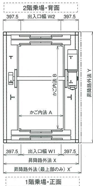
昇降路平面図
