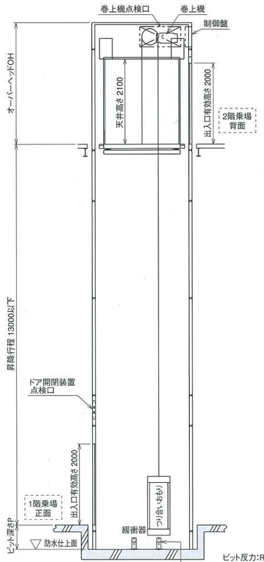
昇降路断面図
