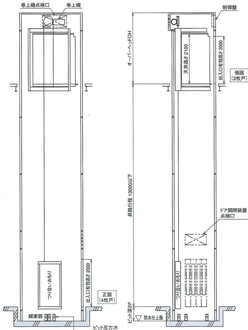
昇降路断面図
